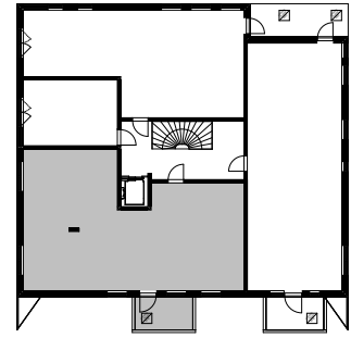
POHJAKAAVIO 1:500
